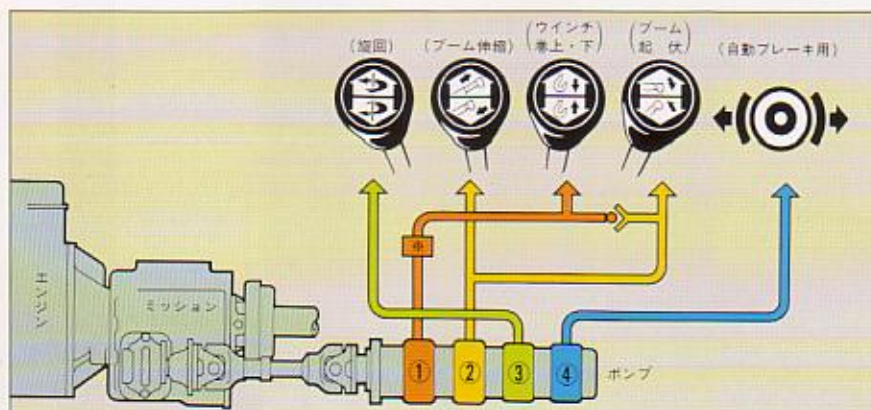
●同時操作を可能にした4連ポンプ(注: ※は圧力補償付流量調整弁を示します)
