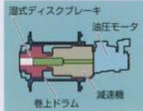
湿式ディスクブレーキ(Opt.)
