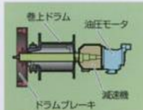
従来のドラムブレーキ
