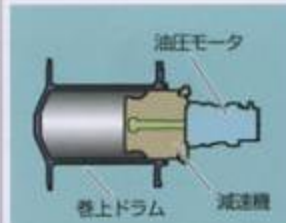
フリーフォールレスウインチ(Std.)
